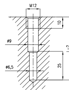
ROZMĚROVÝ NÁKRES VÝVRTU PRO UPEVNĚNÍ SNÍMAČE
